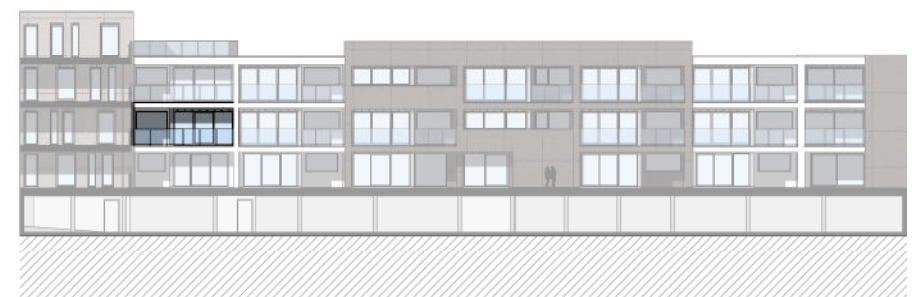
ACHTERGEVEL
